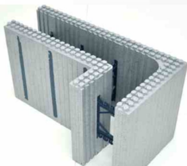
90°veidnis(kreisais)
