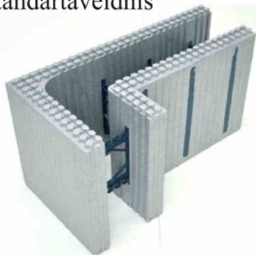
90°veidnis(labais)
