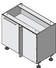
GSP_T_L STŪRA GRĪDAS SKAPIS (LABAIS) 1 PĀRLIEKAMS PLAUKTS W 1000mm (IISO) H = 720mm
