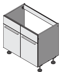
GIZ_2DF IZLIETNES SKAPIS BEZ PLAUKTIEM W 408 - 900mm H = 720mm
