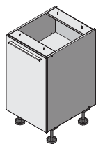
G1D_K/L VERĀMS GRĪDAS SKAPIS (LABAIS/KREISAIS) 2 PĀRLIEKAMI PLAUKTI W 204 - 600mm H = 720mm
