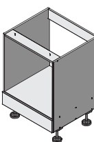
GC GRĪDAS SKAPIS PĀREDZĒTS IEBŪVĒTĀJAI CEPEŠKRĀSNĪ W 600mm H = 720mm
