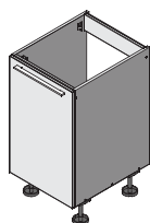
GIZ_1D_K/L IZLIETNES SKAPIS (LABAIS/KREISAIS) BEZ PLAUKTIEM W 400 - 900mm H = 720mm
