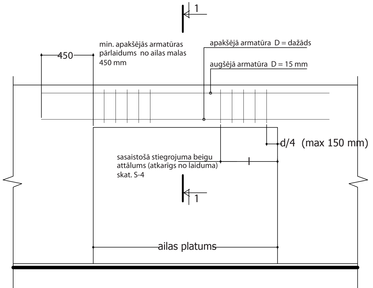
Griezums 1-1
