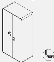
S2 DRĒBJU SKAPIS P/A/Dz - 932/1866/550
