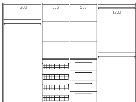
bidāmo durvju ieteicamais novietojums recommended sliding door position
