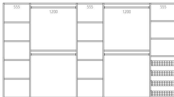
bidāmo durvju ieteicamais novietojums recommended sliding door position
